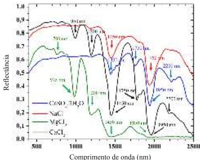
Figura 3. Espectros de refletância dos sais usados no experimento e do gesso ( \text{CaSO}_4 \cdot 2\text{H}_2\text{O} ) usado para tratamento químico das amostras. As posições das principais feições de absorção estão indicadas por setas
