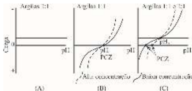
Figura 18. Variação na carga da fração sólida do solo em função do pH e da concentração eletrolítica da solução ambiente para sistemas de carga permanente (A), variável (B) e misto (C)
