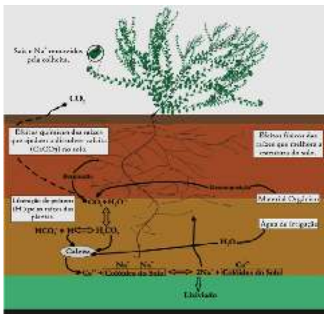
Figura 1. Ilustração dos processos atuantes na fitorremediação de solos afetados por sais: aumento na pressão parcial de \text{CO}_2 na zona radicular, liberação de prótons ( \text{H}^+ ), efeitos físicos das raízes, aumento no teor de matéria orgânica e remoção de sais pela colheita da parte aérea das plantas
