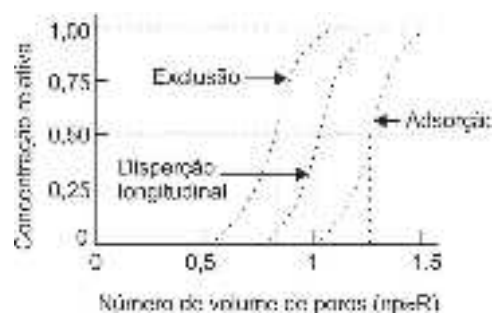
Figura 6. Curvas de efluentes para as situações em que ocorre dispersão-difusão com exclusão, dispersão-difusão apenas e dispersão-difusão com adsorção de um soluto em uma coluna de solo
