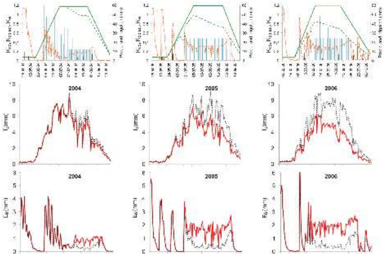
Figura 19. Valores de K_{cb\ pot} (—), K_{cb\ real} (- - - -), E_0 (-----), precipitação (—), e irrigação (—) da cultura do milho usando águas salinas durante as épocas de cultivo de 2004 a 2006, bem como os fluxos de transpiração ( T_p ) e evaporação do solo ( E_s ) diários potenciais (.....) e reais (—) estimados pelo modelo SIMDualKc com as correções para a salinidade
