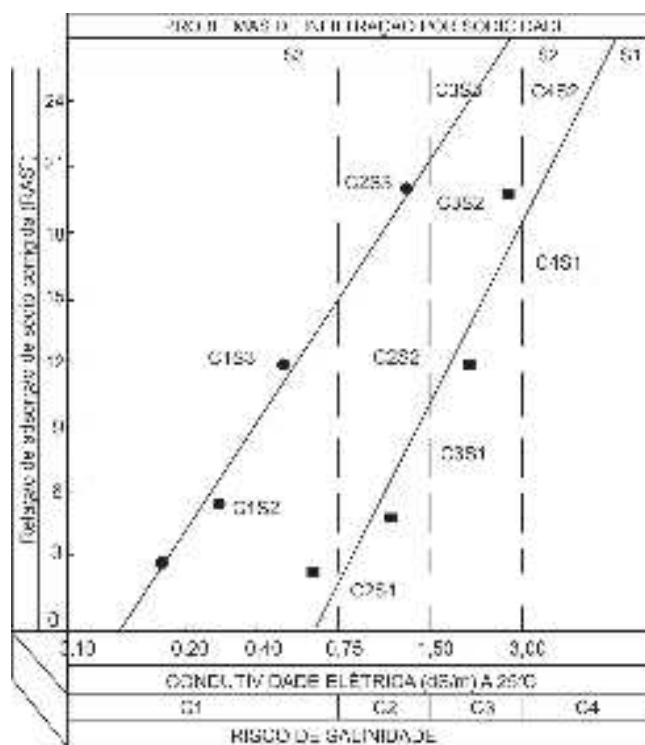
Figura 2. Diagrama aproximado de classes de água para irrigação
