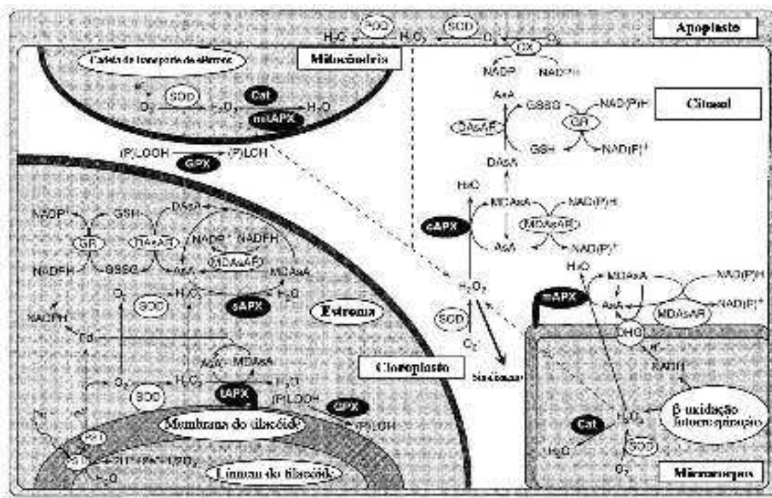
Figura 21. Esquema mostrando as principais organelas e sítios celulares, bem como os componentes metabólicos envolvidos com os processos de produção e de remoção de EROs na célula vegetal. AsA (ascorbato reduzido); MDAsA (ascorbato oxidado)
