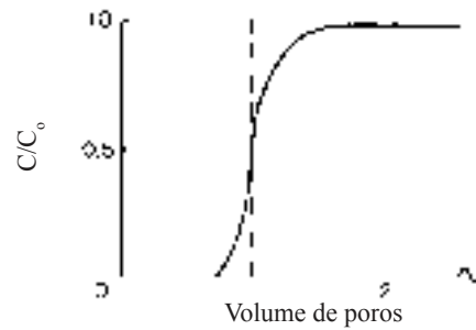
Figura 5. Curva de efluente para escoamento laminar em um tubo
